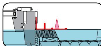
Монтаж на глубине посадки 0 см
