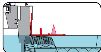
Монтаж на глубине посадки +3 см
